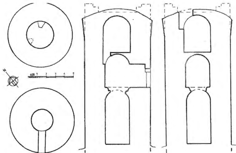
Castell d'Almenara. Plantes i seccions de la torre, amb una indicació de l'enderroc de la part superior abans de la restauració (planimetria: J. R. González, segons dibuix del projecte de J. Fresquet) → Catalunya Romànica , vol. XXIV, pàg. 516 (el Pilar d'Almenara pertany al municipi d'Agramunt)
